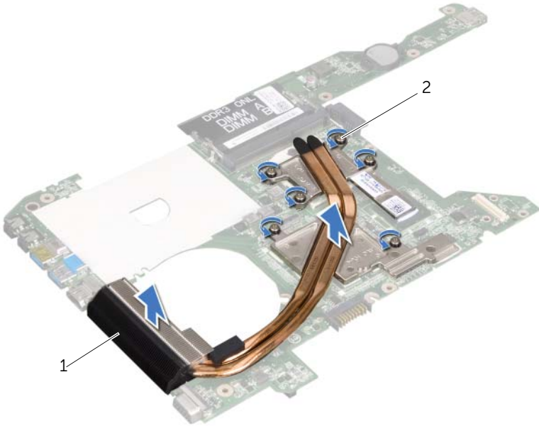
1 프로세서 방열판
